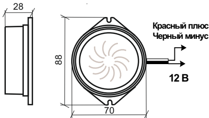
Рис.1. Габаритные и установочные размеры
