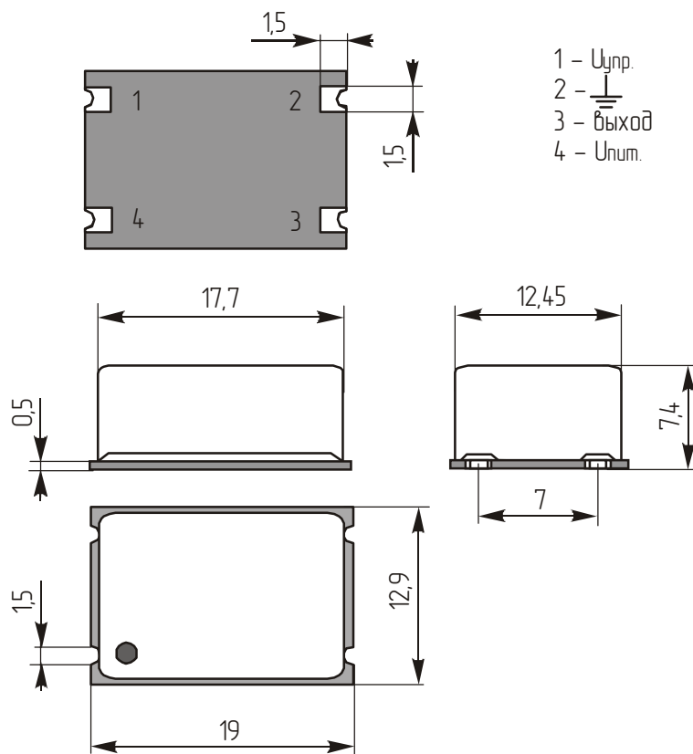
Внешний вид и габаритные размеры (мм)
