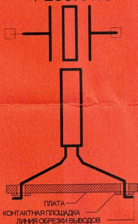
КВАРЦЕВЫЙ РЕЗОНАТОР
