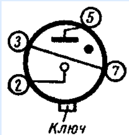
Цоколевка лампы СГ4С
