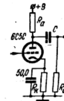
Рис. 471. Схема применения лампы 6С5С в качестве усилителя напряжения низкой частоты на сопротивлениях.
