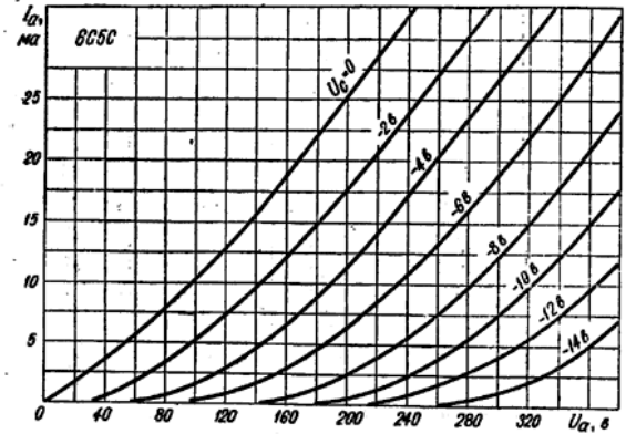
Рис. 474. Упорядоченные характеристики зависимости тока анода от напряжения на аноде.
