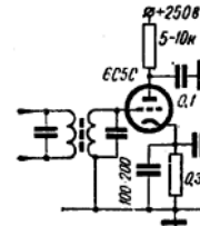
Рис. 472. Схема применения лампы 6С5С в качестве катодного детектора.
