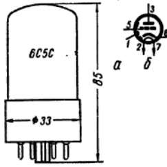
Рис. 470. Лампа 6С5С: а — основные размеры; б — схематическое изображение; 1 — внутренний накал; 2 и 7 — подогреватель (накал); 3 — анод; 4 — сетка; 5 — катод.
