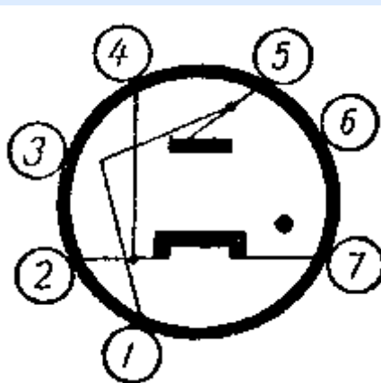
Цоколевка лампы СГ1П
