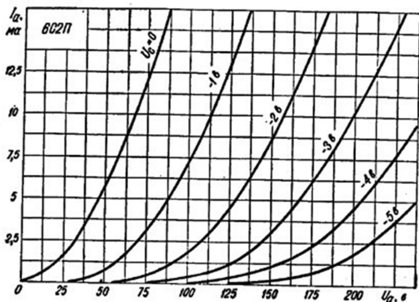
Усредненные характеристики зависимости тока анода от напряжения на аноде.
