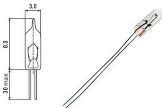
СМН-9-60-2
