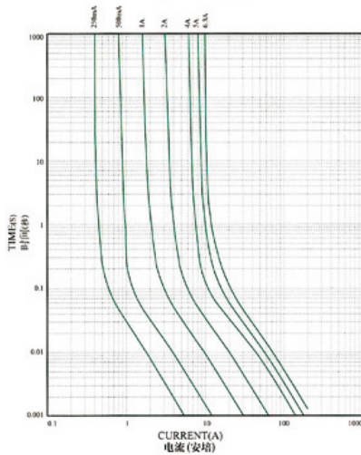
I-T CHARACTERISTICS CURVE 电流-时间曲线图
