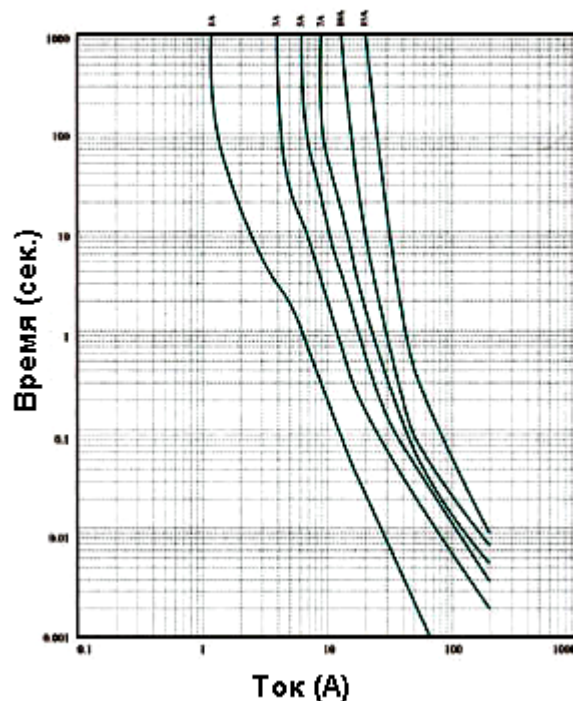
Токовременная зависимость
