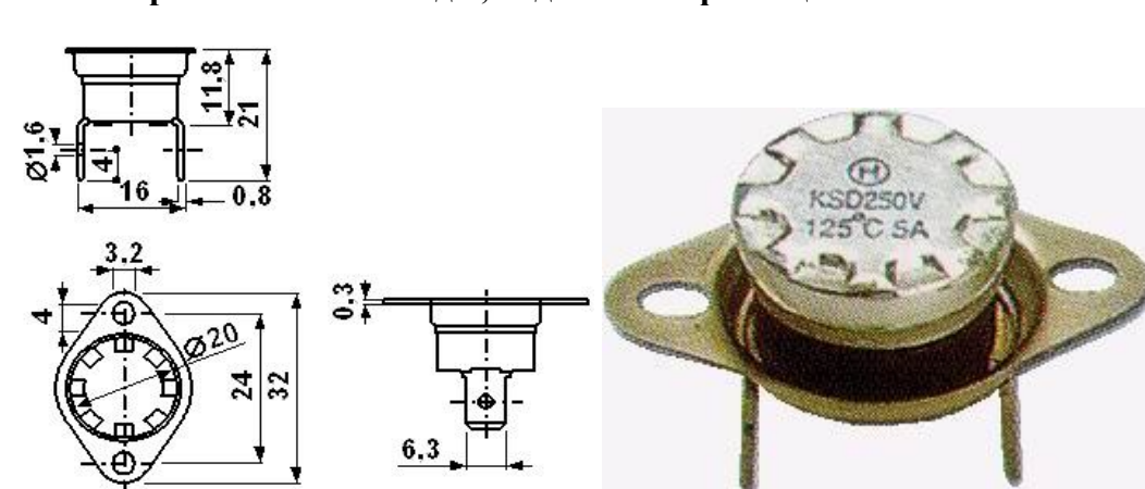
Термостат KSD-F01 серия LBVL вертикальные выводы, подвижный фланец
