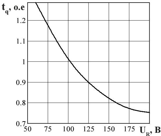
Рисунок 13 - Зависимость времени выключения t_q (о.е.) от обратного напряжения U_R при максимальной температуре перехода T_{jm} = 125 \text{ } ^\circ\text{C} ; I_T = I_{T(AV)} ; (di/dt)_f = 5 \text{ А/мкс} ; dU_D/dt = 50 \text{ В/мкс} ; U_D = 0,67 U_{DRM}
