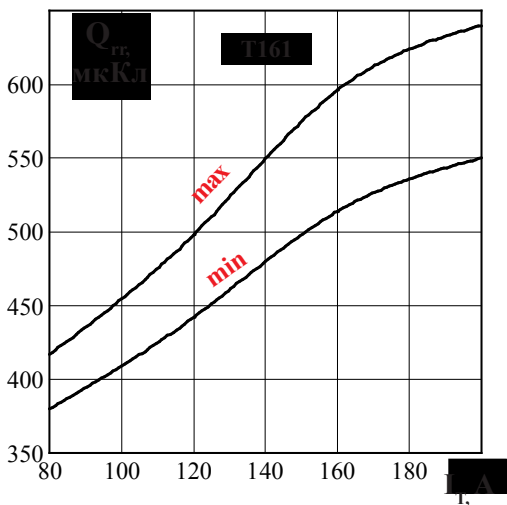
Рисунок 13 - Зависимость заряда восстановления Q_{rr} от тока I_T при U_R = 100\text{ В} ; T_{jm} = 125^\circ\text{C} ; (di/dt)_\rho = 5\text{ А/мкс}
