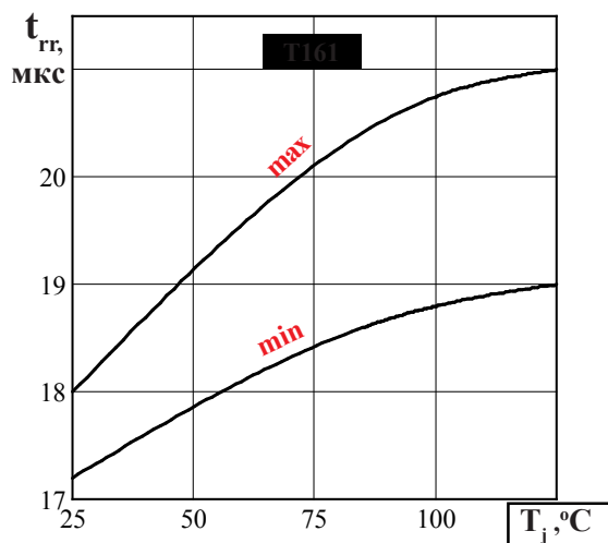
Рисунок 12 - Зависимость времени обратного во- сстановления t_{rr} от температуры структуры T_j при U_R = 100\text{ В} ; I_T = I_{TAVM} ; (di/dt)_\rho = 5\text{ А/мкс}
