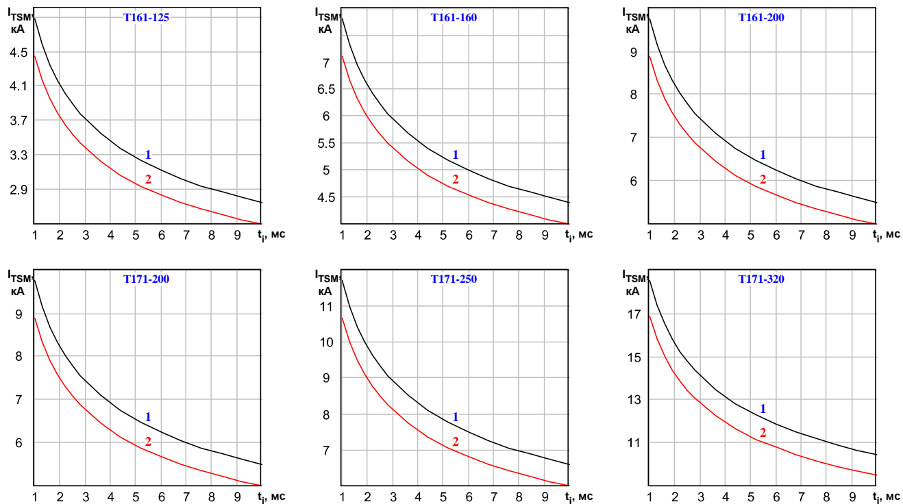
Рисунок 4: Зависимость допустимой амплитуды ударного тока в открытом состоянии I_{TSM} от длительности импульса тока t_i при исходной температуре структуры T_j=25\text{ }^\circ\text{C} (1) и максимально допустимой температуре перехода T_{jm} (2).
