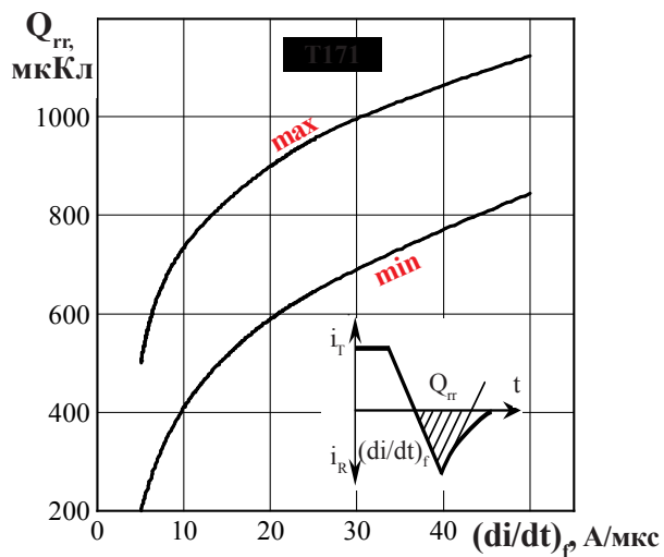
Рисунок 10 - Зависимость заряда восстановления Q_{rr} от скорости спада тока (di/dt)_\rho в открытом состоянии при T_{jm} = 125^\circ\text{C} ; U_R = 100\text{ В} ; I_T = I_{TAVM} .
