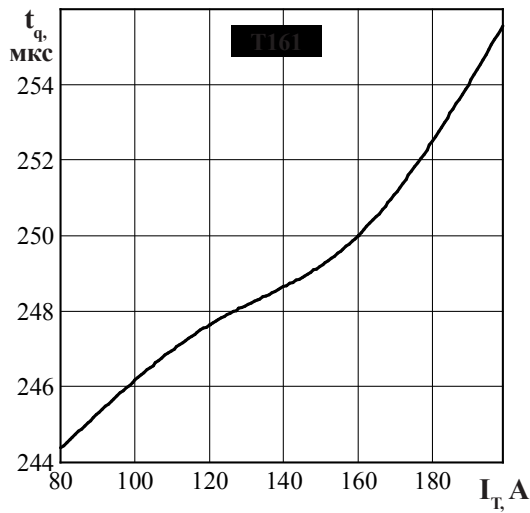
Рисунок 18 - Зависимость времени выключения t_q от среднего тока в открытом состоянии I_T при T_{jm} = 125\text{ }^\circ\text{C} ; U_R = 100\text{ В} ; (di/dt)_f = 5\text{ А/мкс} ; dU_D/dt = 50\text{ В/мкс}
