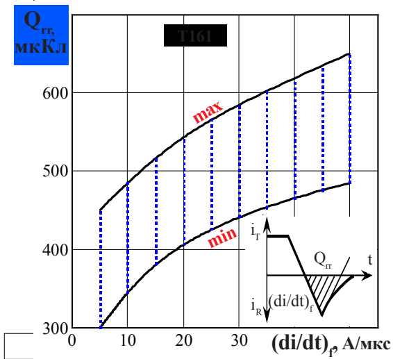
Рисунок 10 - Зависимость заряда восстановления Q_{rr} от скорости спада тока (di/dt)_\rho в открытом состоянии при T_{jm} = 125^\circ\text{C} ; U_R = 100\text{ В} ; I_T = I_{TAVM} .
