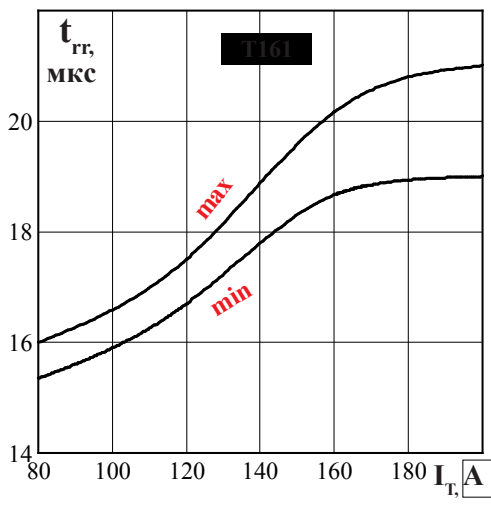
Рисунок 14 - Зависимость времени обратного во- сстановления t_{rr} от тока I_T при U_R = 100\text{ В} ; T_{jm} = 125^\circ\text{C} ; (di/dt)_\rho = 5\text{ А/мкс}
