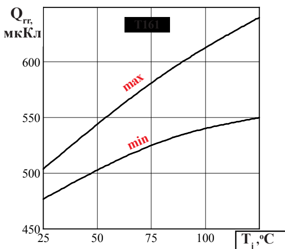
- Зависимость заряда восстановления Q_{rr} от температуры структуры T_j при U_R = 100\text{ В} ; I_T = I_{TAVM} ; (di/dt)_\rho = 5\text{ А/мкс}
