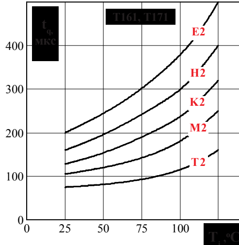
Рисунок 15 - Зависимость времени обратного во- сстановления t_q от температуры структуры T_j при I_T = I_{TAVM} ; U_R = 100\text{ В} ; (di/dt)_\rho = 5\text{ А/мкс} ; d_{T161} = 10\text{ мм}
