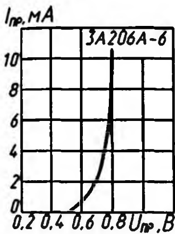
Зависимость прямого тока от напряжения
