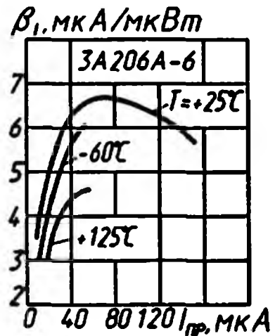
Зависимости чувствительности по току от тока
