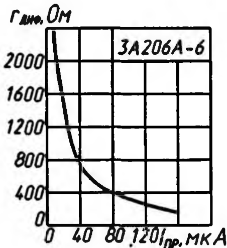
Зависимость дифференциального сопротивления от тока
