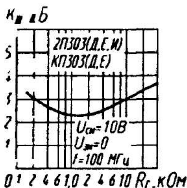
Зависимость коэффициента шума от сопротивления генератора
