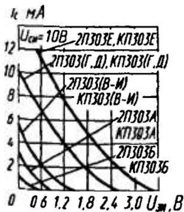
Проходные характеристики
