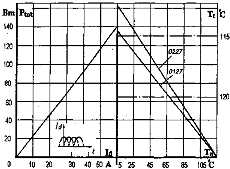
Рис. 2. 26.* Зависимость допустимой суммарной рассеиваемой мощности и допустимого выпрямленного тока трех модулей МТТ4/3 - 63 на охладителях O127 и O227 от температуры окружающей среды и температуры корпуса при естественном охлаждении
