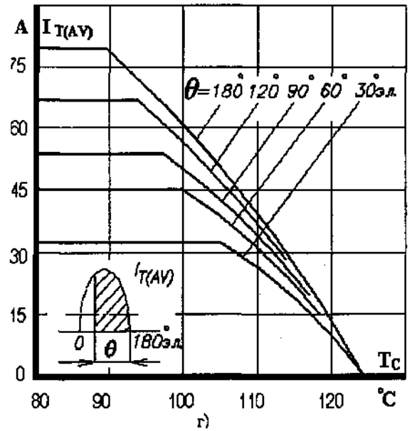
Рис. 2. 3. Зависимость допустимого среднего тока синусоидальной формы в открытом состоянии I_{T(AV)} , частотой 50 Гц, от температуры корпуса T_c при различных углах проводимости:
