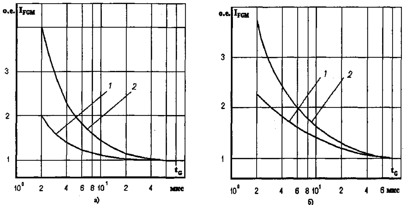
Рис. 2.14. Зависимость отпирающего импульсного тока управления I_{GSM} от длительности управляющего импульса t_G при температуре перехода T_j = 25 °С (1) и минимально допустимой температуре T_{jmin} (2), U_D = 12 В
