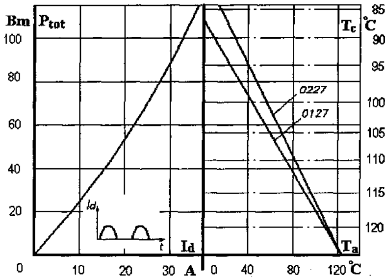
Рис. 2. 21.* Зависимость допустимой суммарной рассеиваемой мощности и допустимого выпрямленного тока одного модуля МТТ4/3 - 40 на охладителях О127 и О227 от температуры окружающей среды и температуры корпуса при естественном охлаждении
