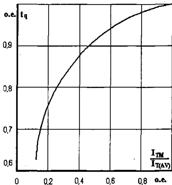
Рис. 2. 9. Зависимость времени выключения t_q от амплитуды предшествующего тока в открытом состоянии I_{TM}/I_{T(AV)} при T_{jm} = 125\text{ }^\circ\text{C} , (di_T/dt)_f = 5\text{ А/мкс} , dU_D/dt = 50\text{ В/мкс} , U_D = 0,67U_{DRM} , U_R = 100\text{ В}
