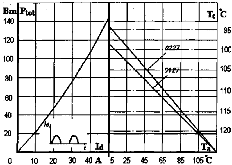
Рис. 2. 24.* Зависимость допустимой суммарной рассеиваемой мощности и допустимого выпрямленного тока одного модуля МТТ4/3 - 63 на охладителях O127 и O227 от температуры окружающей среды и температуры корпуса при естественном охлаждении
