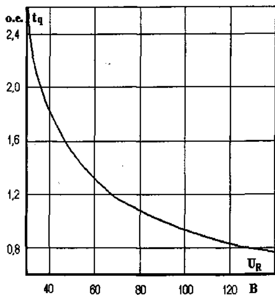
Рис. 2. 8. Зависимость времени выключения t_q от обратного напряжения U_R при максимальной температуре перехода T_{jm} = 125\text{ }^\circ\text{C} , I_{TM} = I_{T(AV)} , di_T/dt = 5\text{ А/мкс} , dU_D/dt = 50\text{ В/мкс} , U_D = 0,67U_{DRM}
