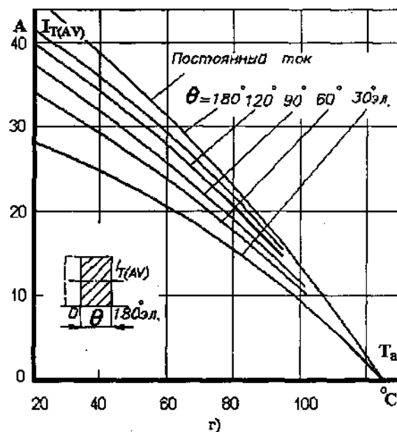
Рис. 2. 16. Зависимость допустимого среднего тока в открытом состоянии I_{T(AV)} прямоугольной формы частотой 50 Гц от температуры окружающей среды T_a при различных углах проводимости и естественном охлаждении на охладителе О127: *
