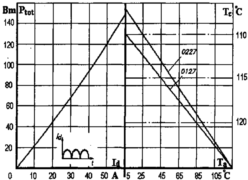
Рис. 2. 25.* Зависимость допустимой суммарной рассеиваемой мощности и допустимого выпрямленного тока двух модулей МТТ4/3 - 63 на охладителях O127 и O227 от температуры окружающей среды и температуры корпуса при естественном охлаждении
