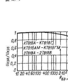
Зависимость относительного напряжения коллектор-эмиттер от сопротивления база-эмиттер.
