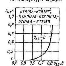
Входная характеристика
