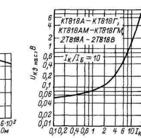
Зависимость напряжения насыщения коллектор-эмиттер от тока коллектора.
