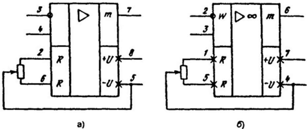
Схемы балансировки К140УД8 (а) и КР140УД8 (б)
