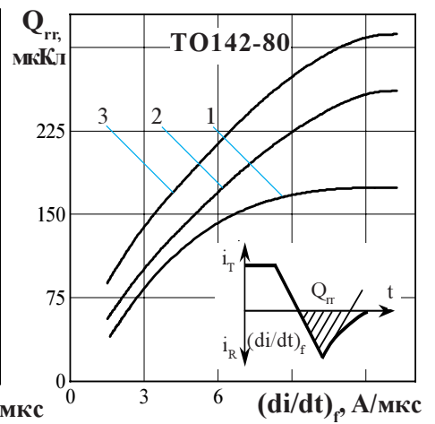
Рисунок 19 - Зависимость заряда восстановления Q_{rr} от скорости спада тока (di/dt)_f в открытом состоянии при температуре перехода T_{jm} = 100\text{ }^\circ\text{C} ; U_{RM} = 100\text{ В} ; I_T = I_{TAVM} .
