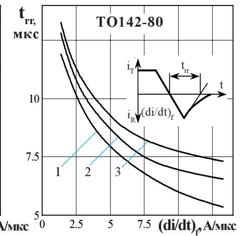
Рисунок 20 - Зависимость времени обратного восстановления t_{rr} от скорости спада тока (di/dt)_f в открытом состоянии при температуре перехода T_{jm} = 100\text{ }^\circ\text{C} , U_R = 100\text{ В} и предшествующем токе открытого состояния I_T = 0,5 I_{TAVM} (1), I_T = I_{TAVM} (2), I_T = 1,5 I_{TAVM} (3).
