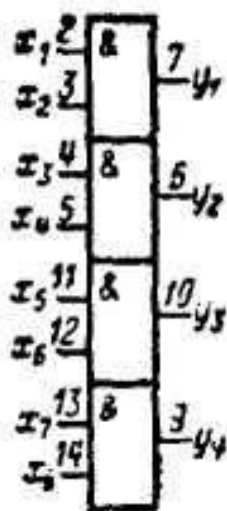
Условное графическое обозначение К172ЛИ1
