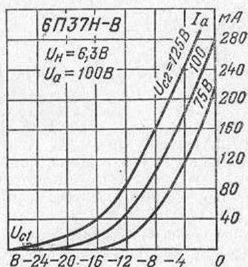
Анодно-сеточные характеристики.
