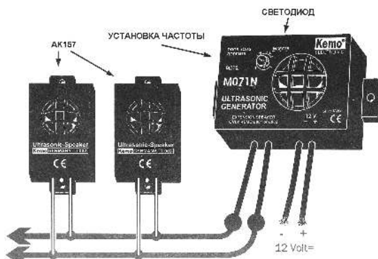
Рис.2 Схема подключений
