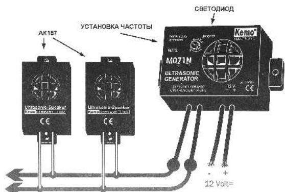
Рис.2 Схема подключений
