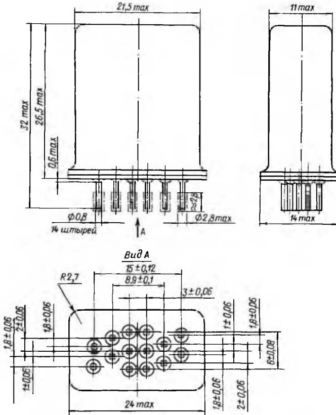
Рис. 2-47. Конструктивные данные реле РЭС53
