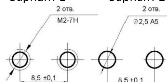
Разметка для крепления Вариант 1 Вариант 2
