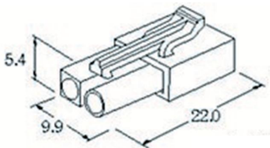
штекер MFC [mini Tamiya]
