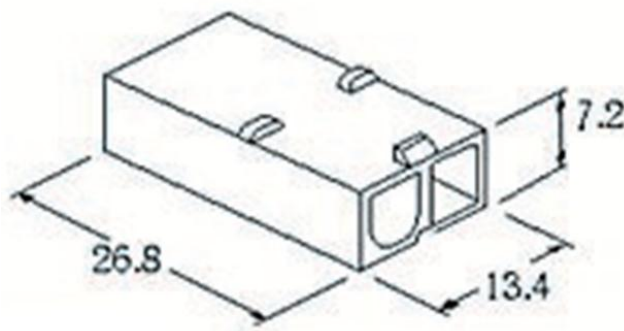
гнездо MFA [Tamiya F]
